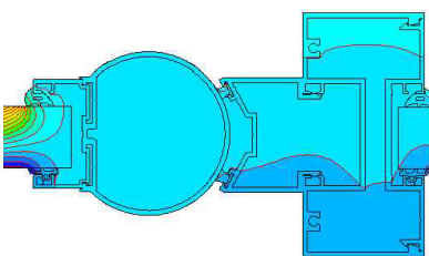
GT55 NI THERMAL PROFILE
